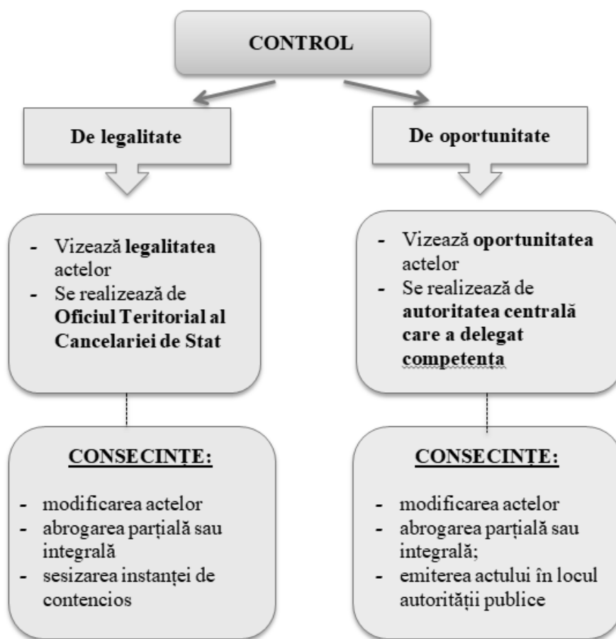
Figura 3.5 Controlul administrativ
